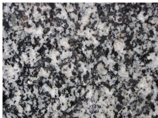
Diorita
