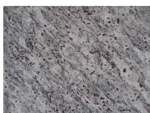
Gneis granatífero
