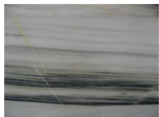
Mármol veteadado
