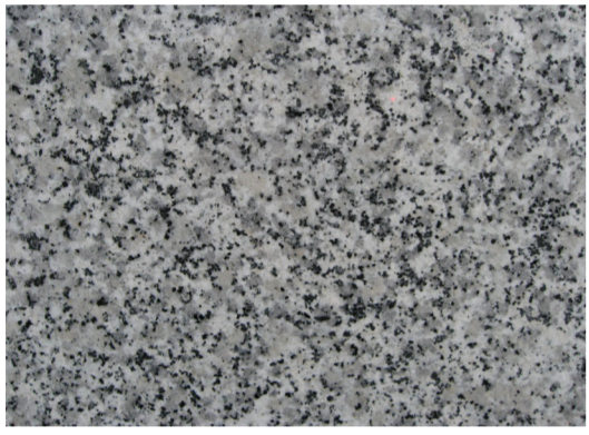
Granito gris
