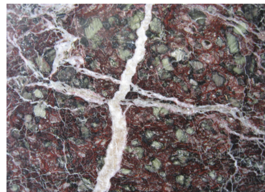
Peridotita serpentinizada
