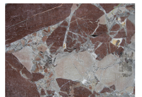
Mármol cataclástico
